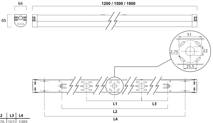
START Batten 1200 /1500 /1800
